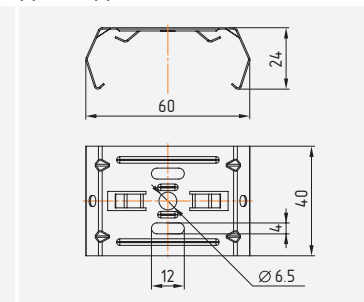
Скоба для монтажа на поверхность (в комплекте)
