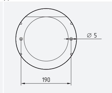
Крепление на опорную поверхность.
