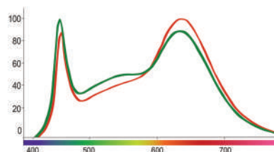
Спектр LED: • томатов и • огурцов
