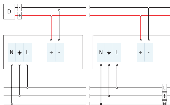
Схема включения интерфейсного датчика освещенности.
