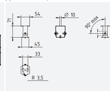
Кронштейн ДСО45/ДСП45 (комплект).
