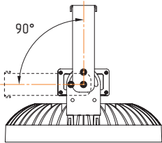
Поворотная лира: схема
