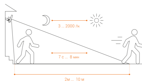
Общая схема
