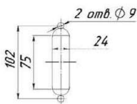
Рис. 2. Разъединитель серии P с передней смещенной рукояткой PC-2, PC-4, PC-6, на номинальный ток 250 А, 400 А и 630 А
