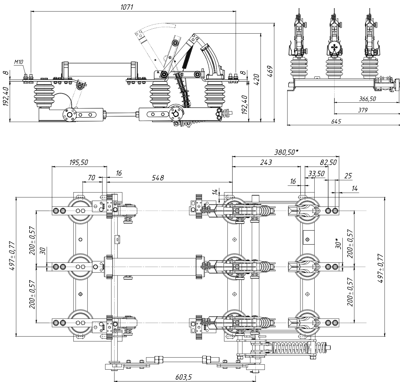
Рис. 3. Выключатель нагрузки автогазовый типа ВНАП-10/630-20-III ПТ 1.2 У2, масса не более 46,5 кг
