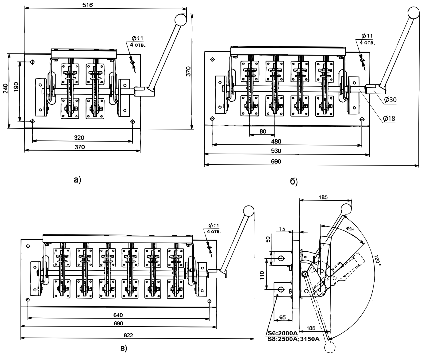
Рис. 52. Разъединитель PE19 с боковой рукояткой, заднего присоединения шин, на изоляционной плите а) PE19-44(45, 46)-12220-00 УХЛЗ, и/п; б) PE19-44(45, 46)-22220-00 УХЛЗ, и/п; в) PE19-44(45, 46)-32220-00 УХЛЗ, и/п
