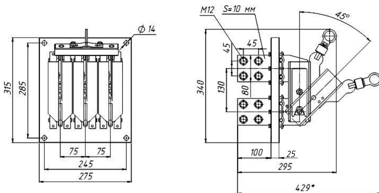
Рис. 56. Разъединитель PE19 с центральным рычагом для управления штангой, на изоляционной плите PE19-49-12290-00 УХЛ3, и/п
