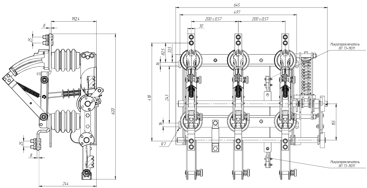
Рис. 22. Выключатель нагрузки автогазовый типа ВНАП-10/630-20-Из У2 с микропереключателем, масса не более 36,5 кг
