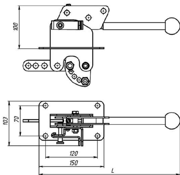
Рис. 26. Привод ПРБД-10
