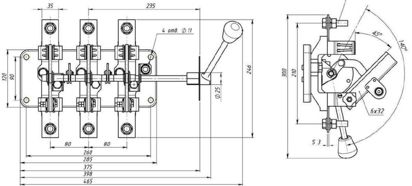
Рис. 5. Разъединитель серии P с боковой рукояткой РБ-6, на номинальный ток 630 А
