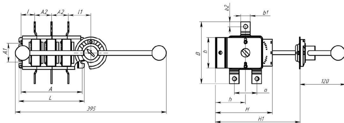
Рис. 17. Выключатель-разъединитель на два направления трехполюсный с передней поворотной ручкой
