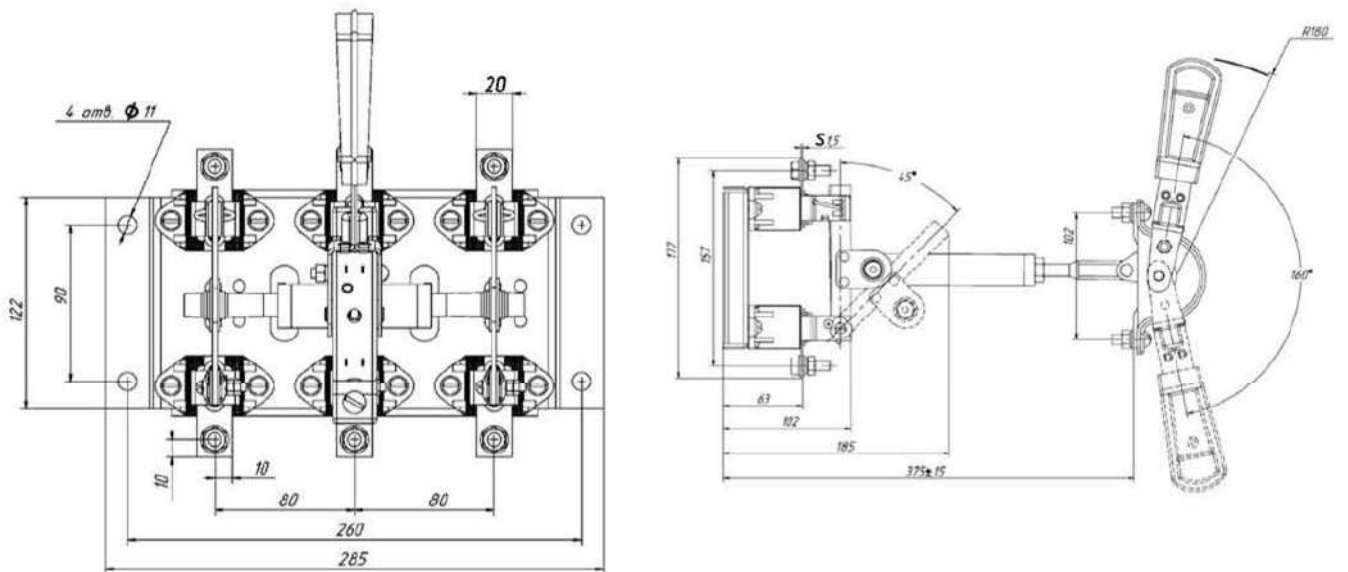
Рис. 6. Разъединитель серии P с центральным приводом РС-1, на номинальный ток 100 А
