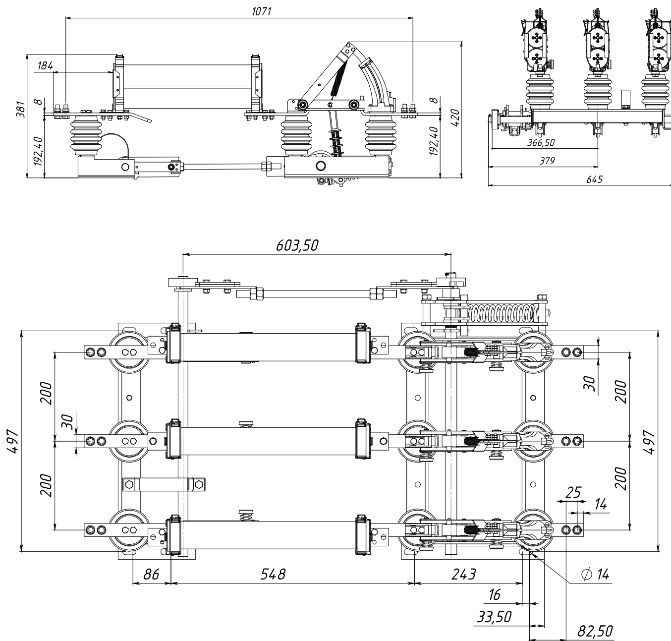
Рис. 6. Выключатель нагрузки автогазовый типа ВНАЛ-10/630-20-III ПТ 1.3 У2, масса не более 47 кг
