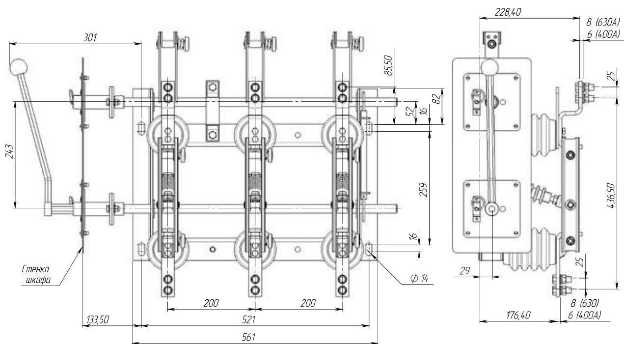
Рис. 6. Разъединитель внутренней установки типа RV3 с левым продольным приводом RV3лр-10/400 (630)-I U2, масса не более 28,5 кг
