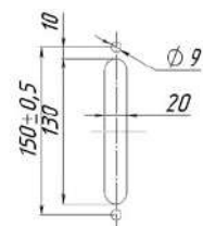
Рис. 12. Разъединитель PE19-39-31140-00 УХЛЗ с передней смещенной рукояткой
