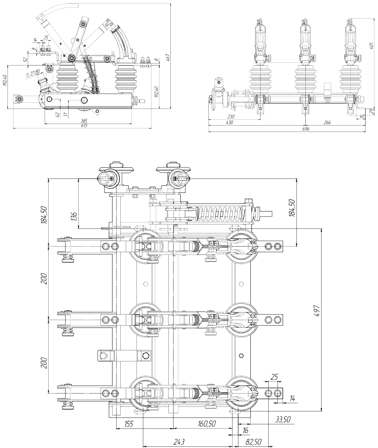
Рис. 25. Выключатель нагрузки автогазовый типа ВНАЛш-10/630-20-ИлзУ2, масса не более 38 кг
