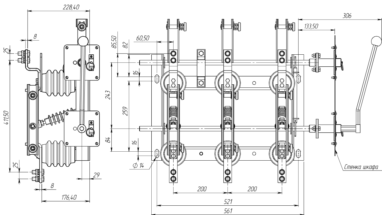
Рис.5. Разъединитель внутренней установки типа RV3 с правым продольным приводом RV3пр-10/630-I U2, масса не более 28,5 кг
