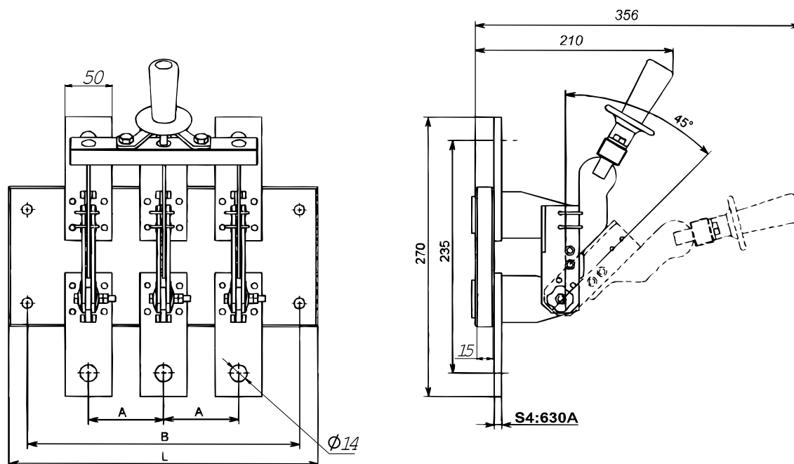
Рис. 13. Разъединитель PE19-39-21170-00 УХЛЗ с рукояткой для полюсного оперирования
