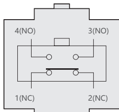
Рис. 1. Расположение контактов
