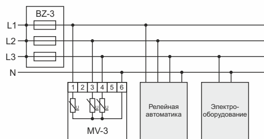
Подключение MV-4
