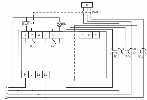
Схема подключения OM-630-2
