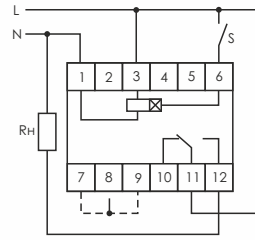
Запуск реле управляющим сигналом
