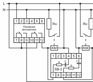
Подключение SB-2
