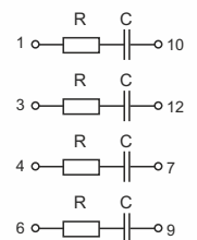
Подключение SB-4
