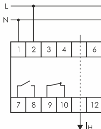
Схема для контроля токов до 50 А
