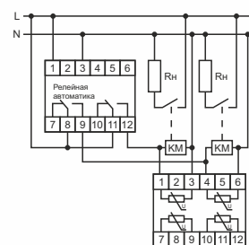
Подключение MV-3
