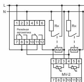
Подключение MV-2
