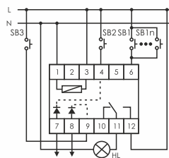
BIS-412
