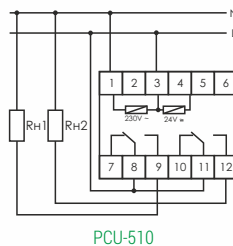
PCU-510
