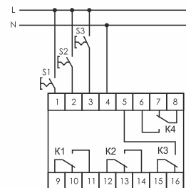
Схема запуска для функции 9
