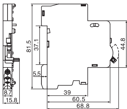
ДК-105 и СК-105
