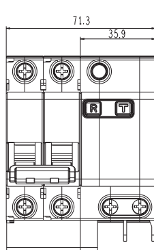
ДИФ-101 2P 63A
