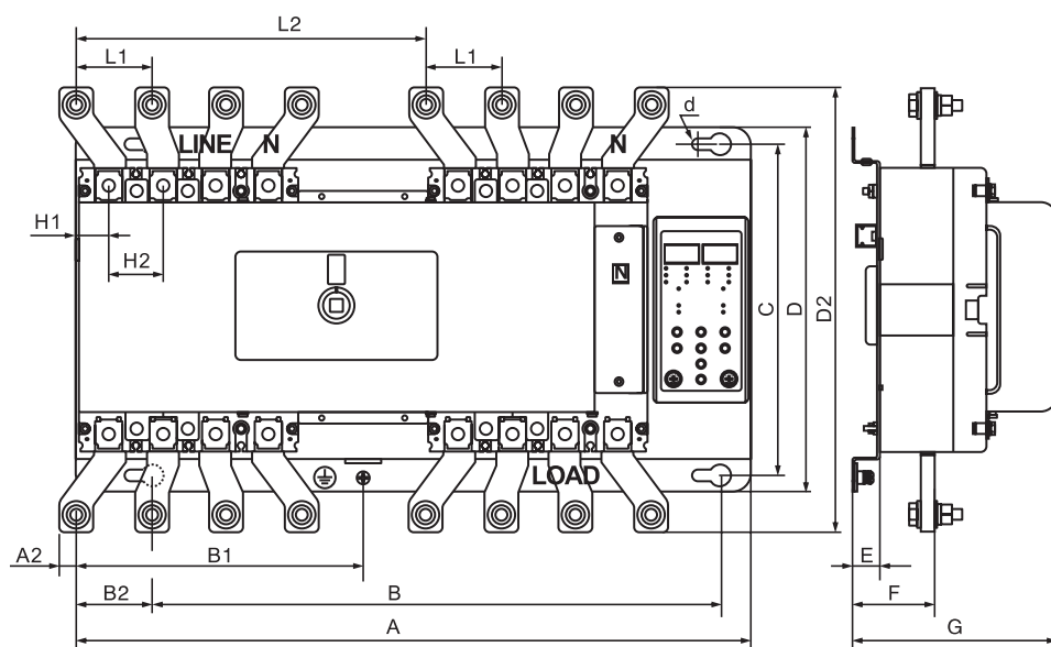
Габаритные размеры ABP-305 (400-630A) 3P/4P со встроенным блоком управления
