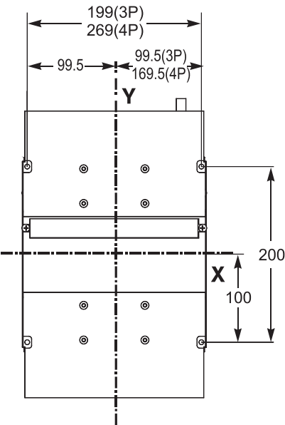
Безопасные установочные расстояния
