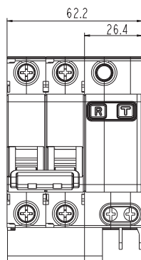
ДИФ-101 2P 32A
