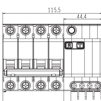
ДИФ-101 4P 32A
