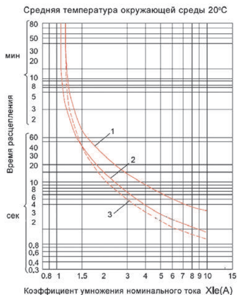
График 1: 3 полюса из «холодного состояния» График 2: 2 полюса (обрыв фазы) из «холодного состояния» График 3: 3 полюса из «горячего состояния»
