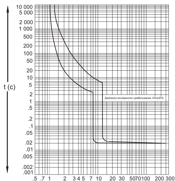
ABP-304
