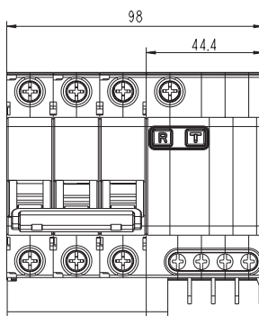
ДИФ-101 3P+N 32A
