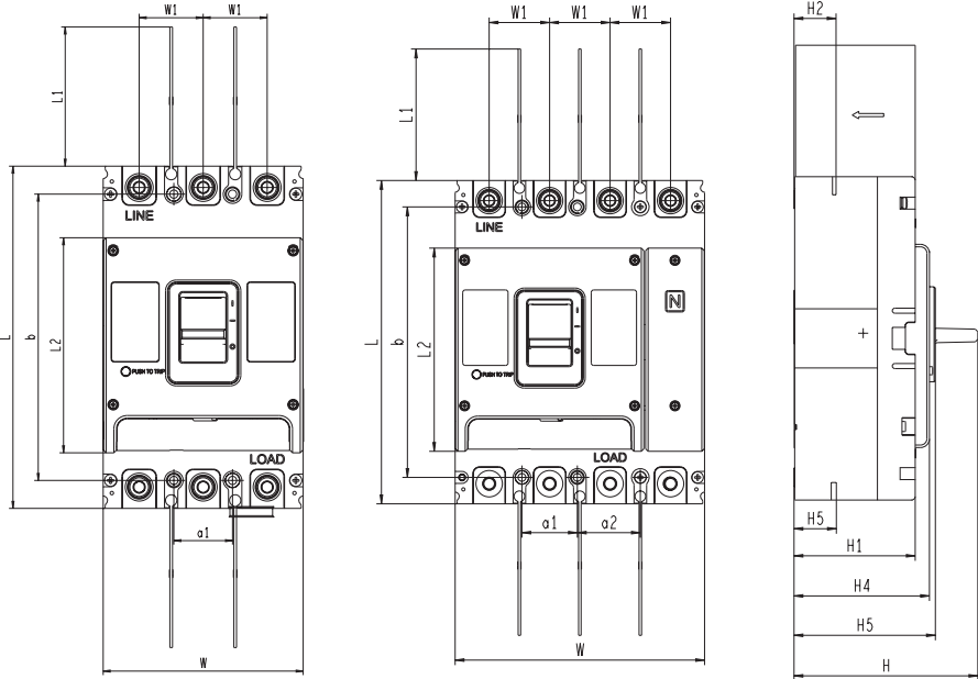
BA-333E / BA-335E / BA-336E
