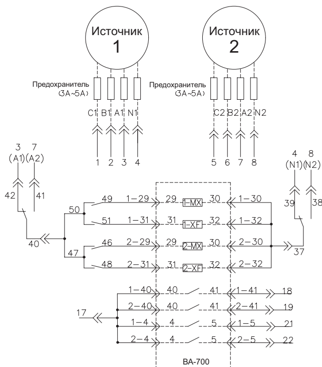
Электрическая схема подключения АВР-701-2
