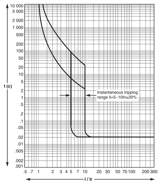
BA-333A (160-250 A)
