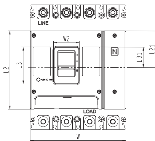
Размеры отверстий фиксированных и съемных панелей аппарата (мм)
