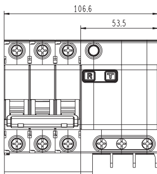
ДИФ-101 3P 63A
