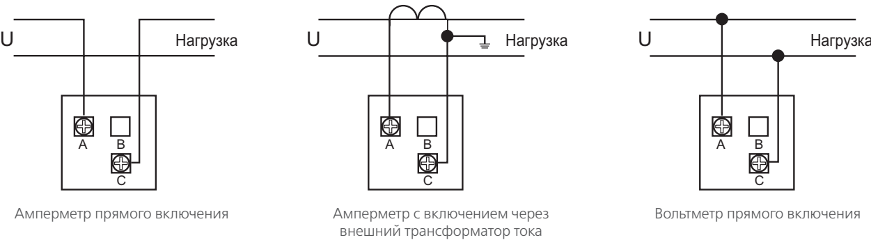
Измерительные приборы переменного тока
