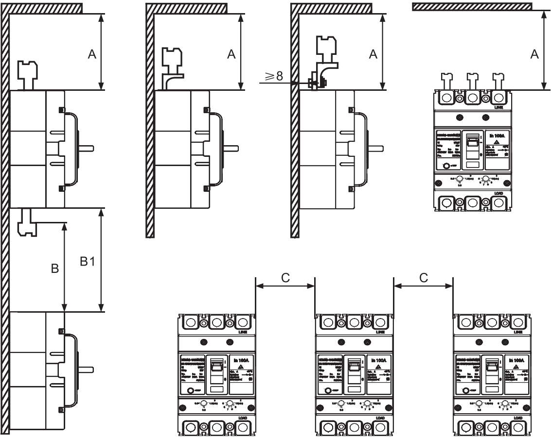
Безопасное расстояние между выключателями
