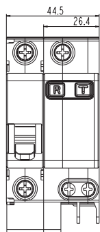
ДИФ-101 1P+N 32A
