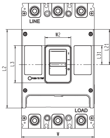
Размеры отверстий фиксированных и съемных панелей аппарата (мм)
