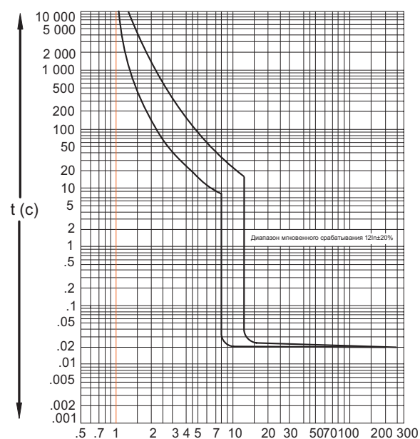
ABP-303
