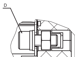
Размер монтажного отверстия клеммной пластины (мм)
