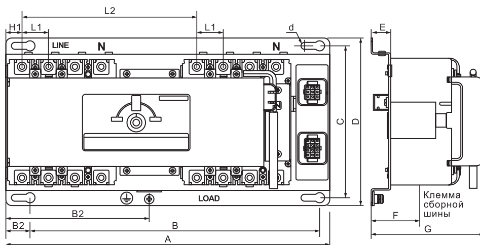
Габаритные размеры ABP-301..304 (10-400A) 3P/4P с выносным блоком управления
