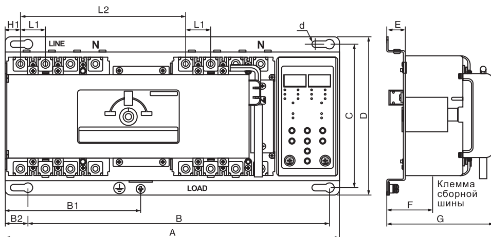
Габаритные размеры ABP-301..304 (10-400A) 3P/4P со встроенным блоком управления
