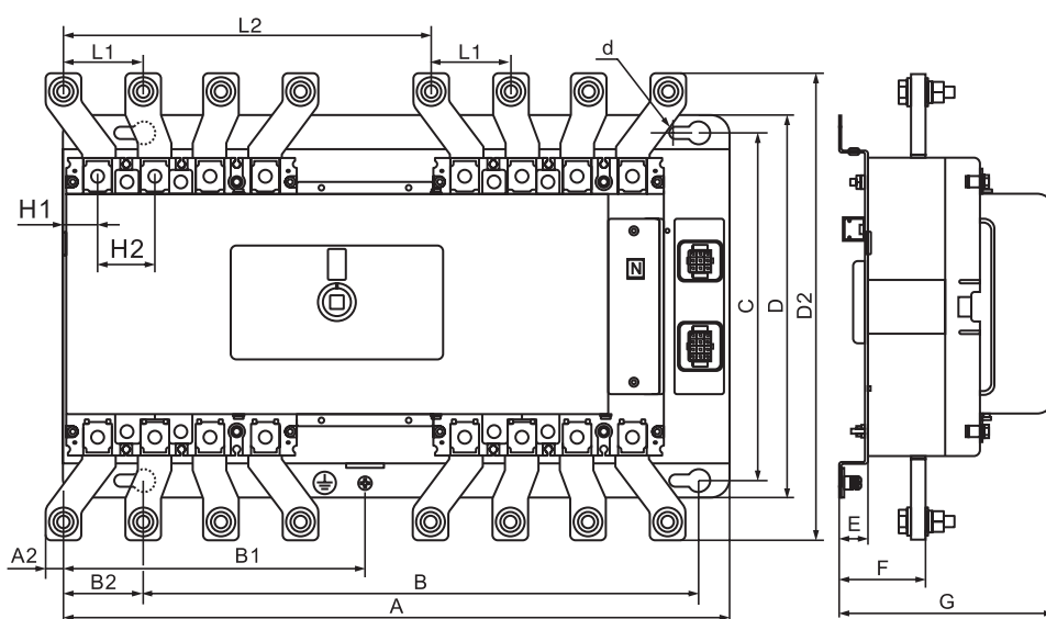
Габаритные размеры ABP-305 (400-630A) 3P/4P с выносным блоком управления
