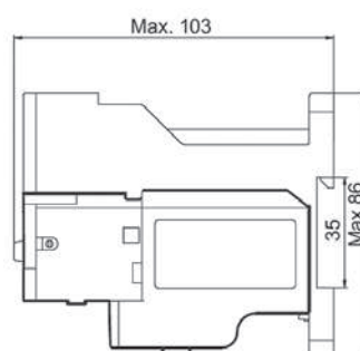
PT-03 для контакторов 25-32 А, независимая установка
