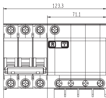
ДИФ-101 3P+N 63A
