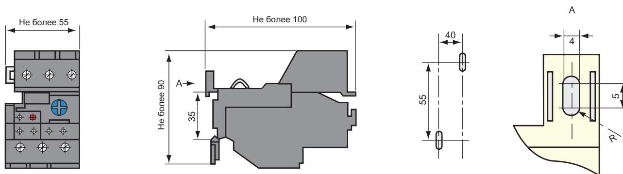
Габаритные и установочные размеры реле тепловых РТ-02-(25-38А) в клеммной колодке КК-02-(25-38А)
