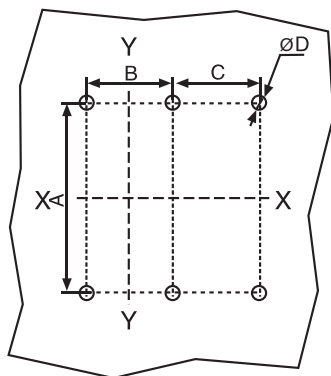
Шаблон для разметки монтажной панели (мм)
