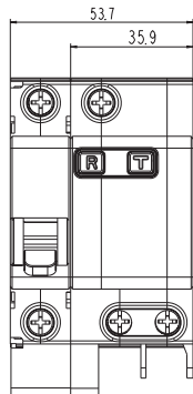
ДИФ-101 2P 63A
