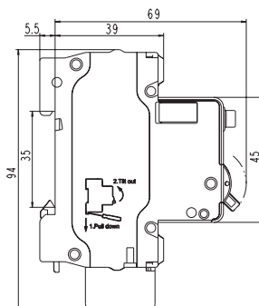
ДИФ-101 3P 32A
