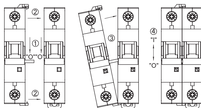
Присоединение независимого расцепителя в отдельном модуле к выключателю проводят в следующей последовательности (см. Руководство по эксплуатации независимого расцепителя)
