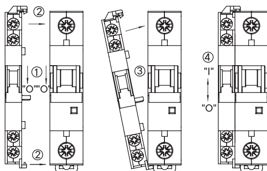
Присоединение модулей со вспомогательными контактами к выключателю или к модулю с независимым расцепителем (см. Руководство по эксплуатации модулей вспомогательных контактов)
