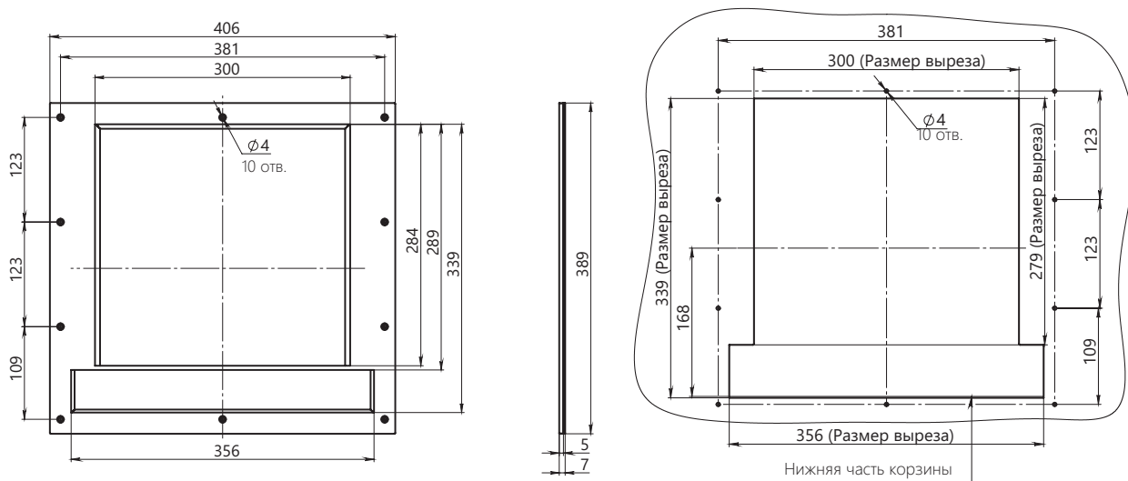
Рамка передней панели выдвижного YON 2500-6300A-UHL3
