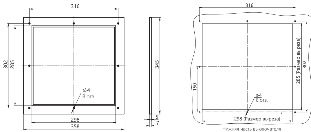
Рамка передней панели стационарного YON 630-6300A-UHL3
