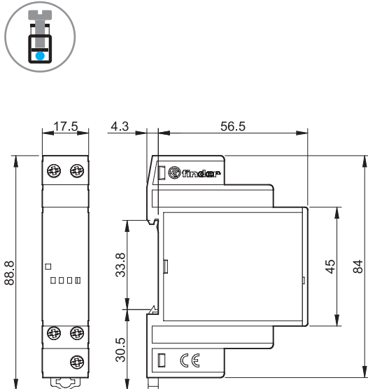
Тип 19.91 (Силовой модуль для модели 11.91) Винтовые клеммы
