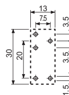
95.13.2 Вид сбоку
