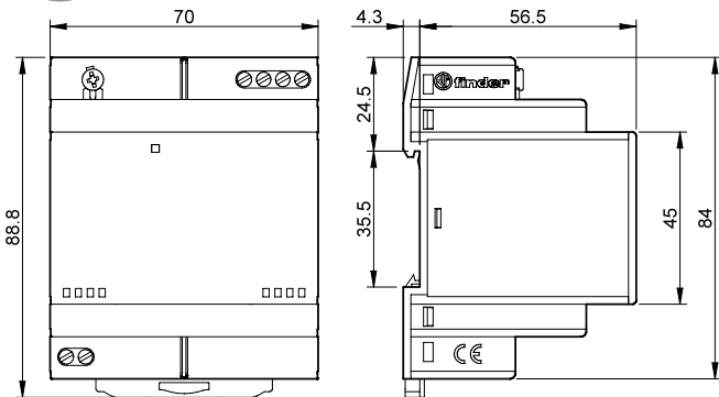
Тип 78.1В Винтовой клеммы
