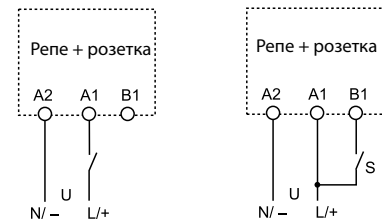
Схема подключения (без сигнала START) Схема подключения (с сигналом START)
