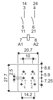
56.42-0300 Вид со стороны выводов
