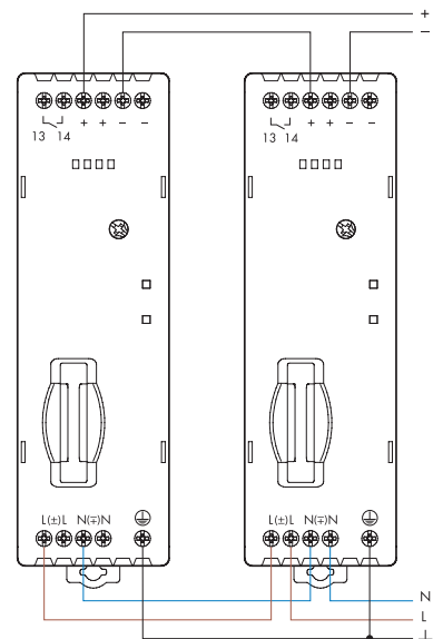
Последовательное подключение
