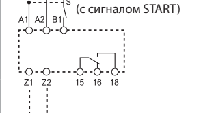
Схема подключения (с сигналом START)
