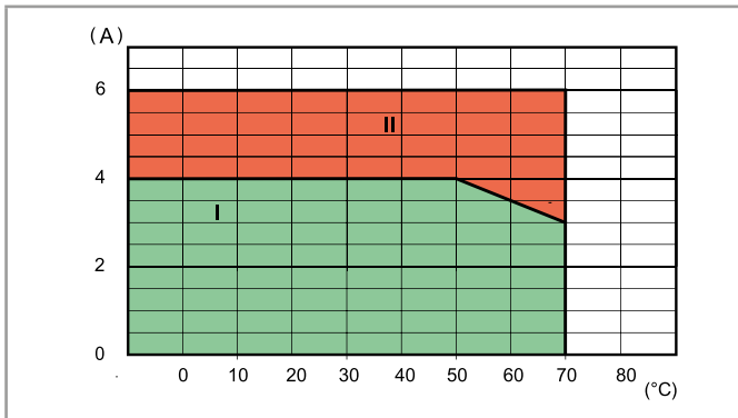
L 39-1 - Зависимость тока выход. цепи DC от температуры 39.xx.x.xxx.9024
