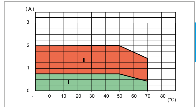
L 39-2 - Зависимость тока выход. цепи AC от температуры 39.xx.x.xxx.8240
