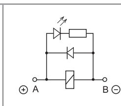
C: Опция 6, 7, 74 Светодиод + диод (DC, полярность положительная для контакта A/A1)
