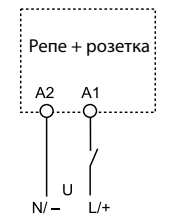
Схема подключения
