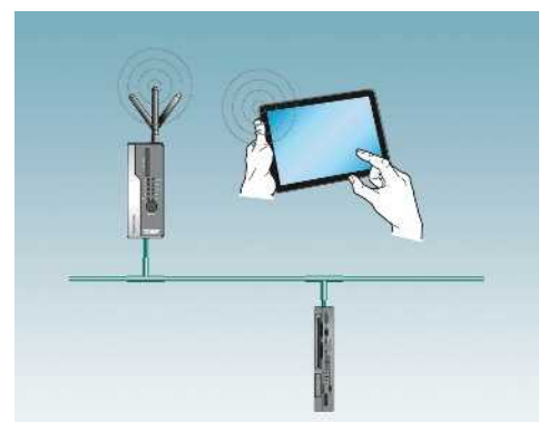
Visu+ mobile на мобильном конечном устройстве посредством точки доступа, с промышленным ПК и веб-сервером в качестве опции
