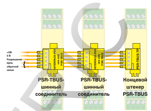
Шинные соединители на DIN-рейке PSR-TBUS осуществляют подключение модулей.
