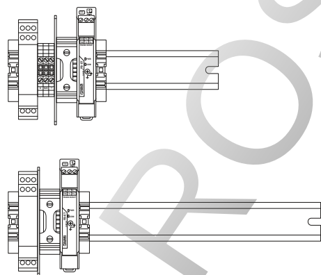
Компоненты несущей шины, сравнение корпусов маленького и большого размера
