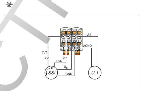
1 SSI-интерфейс для датчика абсолютных значений, 1 аналоговый выход
