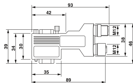
Размерный чертеж SUBCON-PLUS...90X...M12, длинная модель 90°
