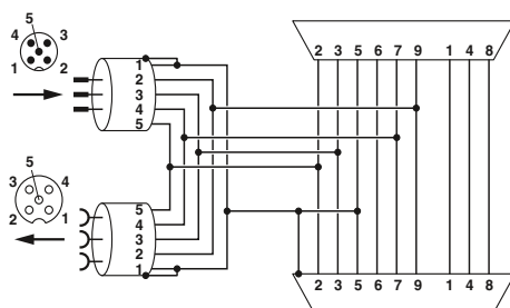
Функциональная схема SUBCON-PLUS-CAN/...M12
