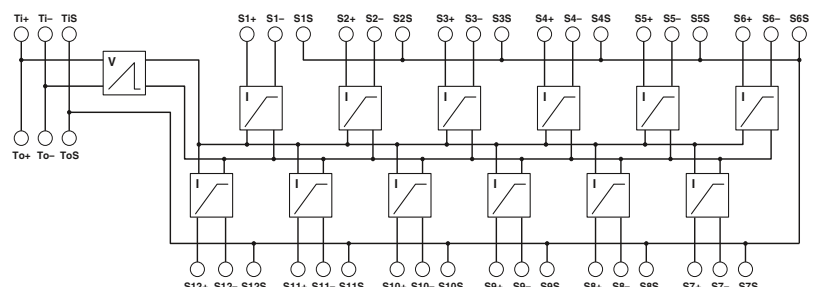
Схема подключения: FB-12SP
