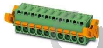
С контрольным отводом и рычагами Lock & Release для фиксации и выталкивания
