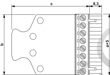
Тип: MSTB 2,5/...-5,08 с CC 2,5/...-G-5,08 P26THR
