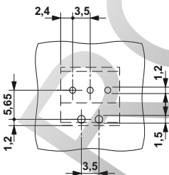
Схема расположения отверстий для MKDSFW 1,5/3-3,5
