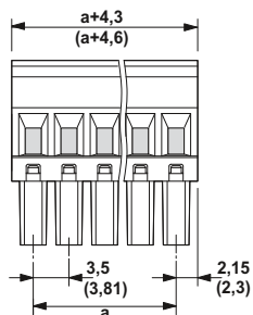
Чертеж
