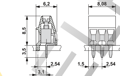
MPT 0,5/...-2,54, количество контактов 2 или 3, см. стр. 83.
