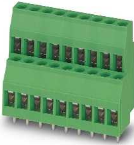
Двухъярусные клеммы для печатных плат, со смещенными ярусами, соединение встык
