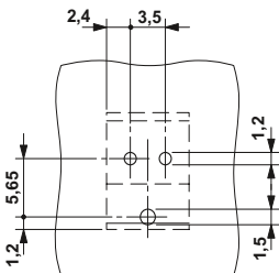
Схема расположения отверстий для MKDSFW 1,5/2-3,5
