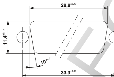
Монтажный вырез согласно DIN 41652-3 для корпусов с толщиной стенки до 2,0 мм PSC 1,5/5..M(-PE) см. стр. 251.
