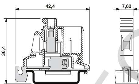
Чертеж
