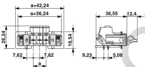
Чертеж
