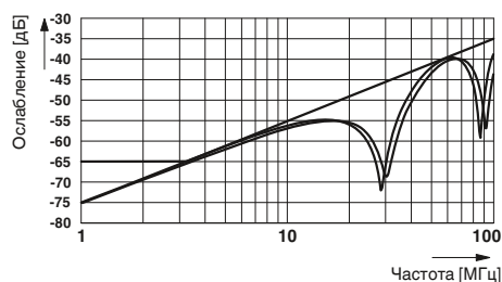
Переходное затухание на ближнем конце для штекера РТРМ с кабелем Ethernet
