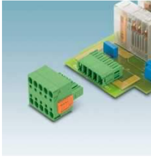
Серия PC 5: штекеры со двоянными пружинными зажимами, до 41 А, шаг 7,62 мм TSPC 5...
