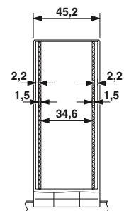
Внутренние размеры корпуса
