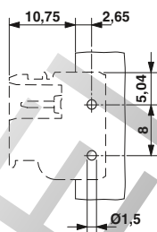
Схема расположения отверстий
