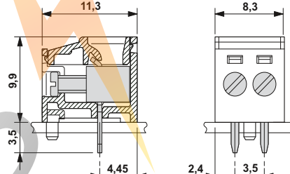
MKDSFW 1,5/2-3,5 (с опорным штифтом), см. стр. 87.
