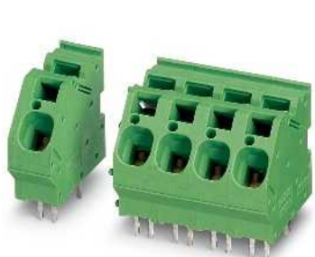
Шаг 10 мм, с контрольным отводом, возможность установки перемычек
