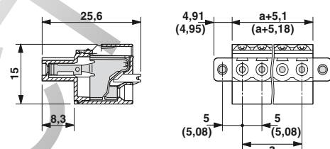
Чертеж
