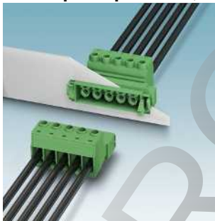
Серия PC 16: инвертированные проходные ответные части, с выводами под пайку и винтовыми зажимами, до 76 А, шаг 10,16 мм DFK-IPC 16...
