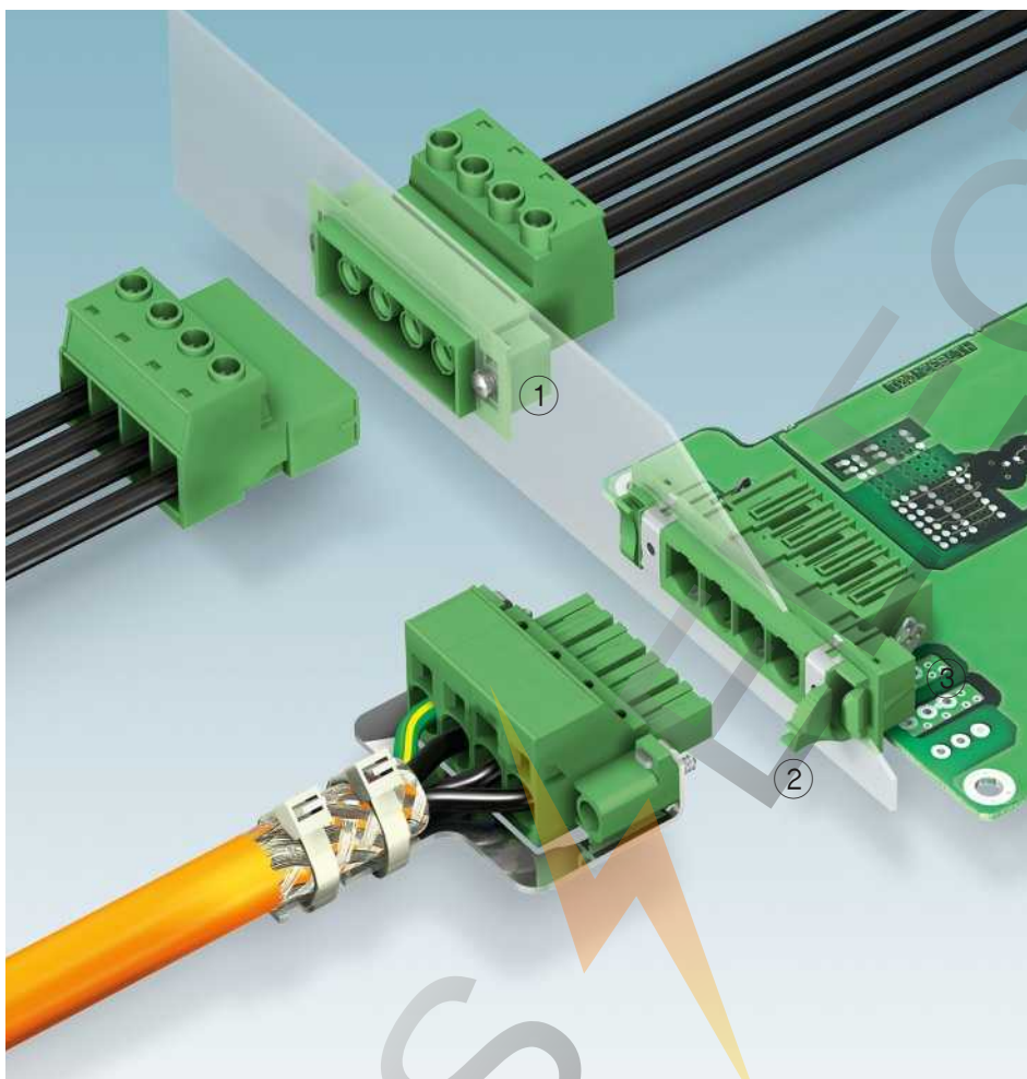
1 Винтовое крепление
