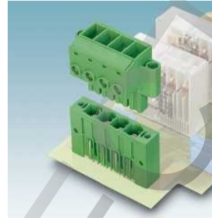
Серия PC 16: штекерная/ответная часть с винтовыми зажимами, до 76 А, шаг 10,16 мм PC 16/...
