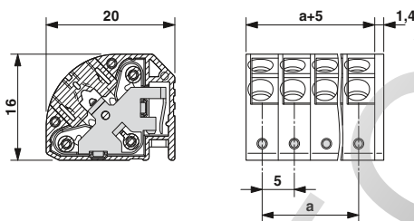
Чертеж
