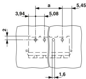
Схема расположения отверстий
