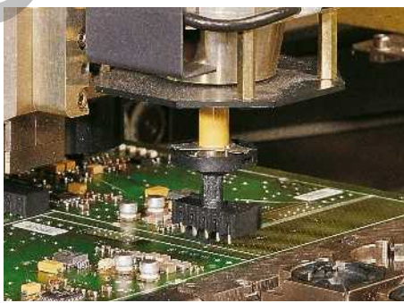
"положить" ("Place") компонент на печатную плату
