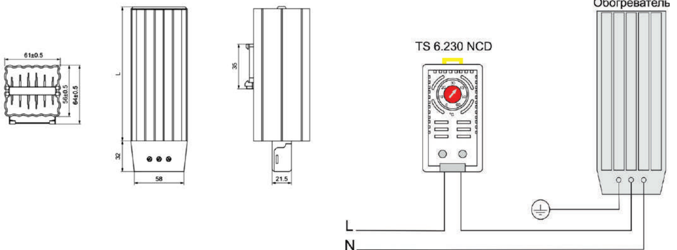
Схемы подключения
