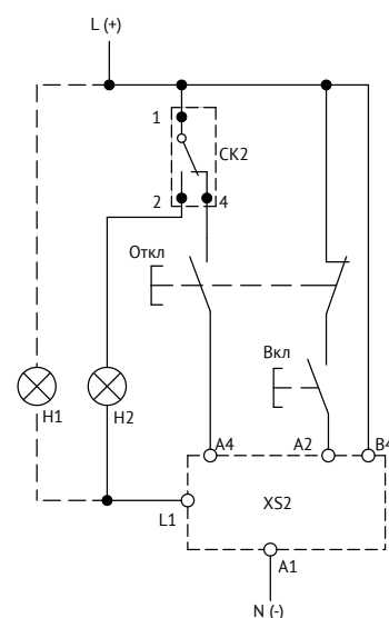
Схема подключения привода с импульсными командами управления без автоматического взвода включающей пружины после срабатывания CK2
