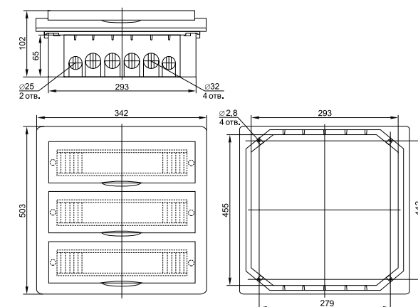
ЩРВ-П-36
