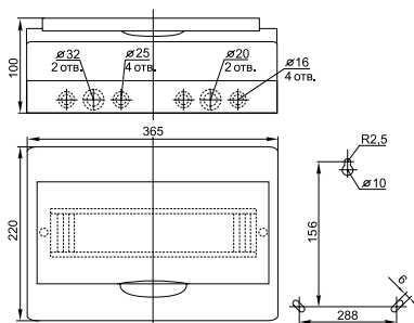
ЩРН-П-18
