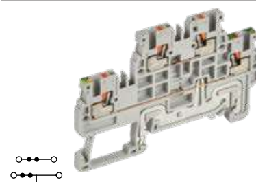
CP-ML-PEN 2 ур. 1,5 мм²
