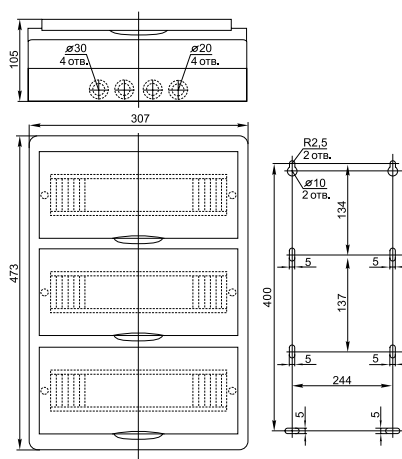
ЩРН-П-36
