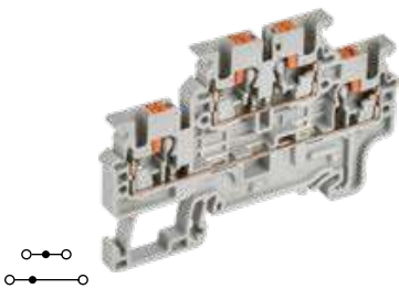
CP-ML 2 ур. 2,5 мм²
