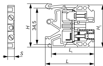
Габаритные размеры
