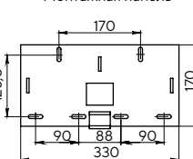
Монтажная панель
