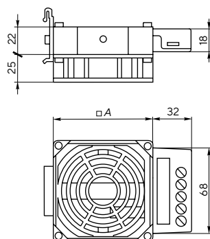
Обогреватель на DIN-рейку (встр. вент.)
