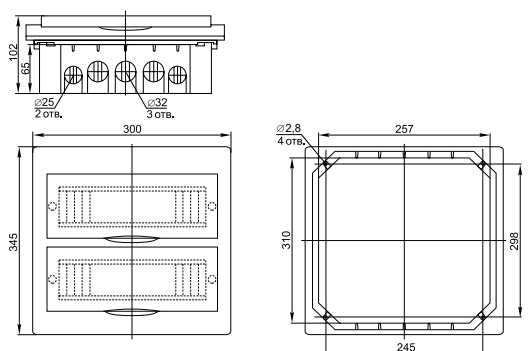
ЩРВ-П-24
