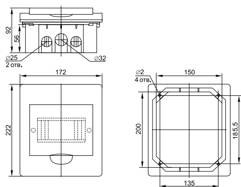
ЩРВ-П-6
