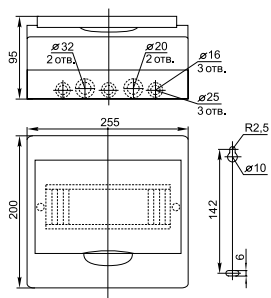
ЩРН-П-12
