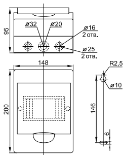
ЩРН-П-6
