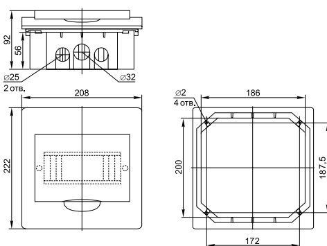
ЩРВ-П-8
