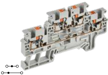
CP-ML 2 ур. 4 мм²
