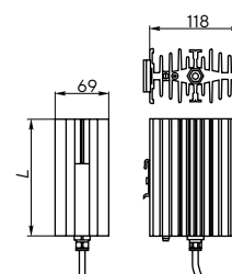
Обогреватель на DIN-рейку
