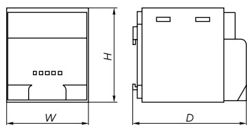
Обогреватель на DIN-рейку в корп. (встр. вент.)
