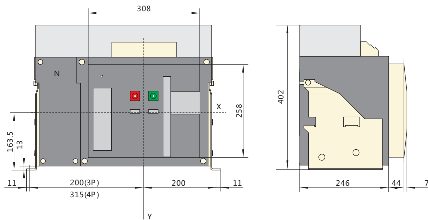
NA8G-3200 стационарное исполнение
