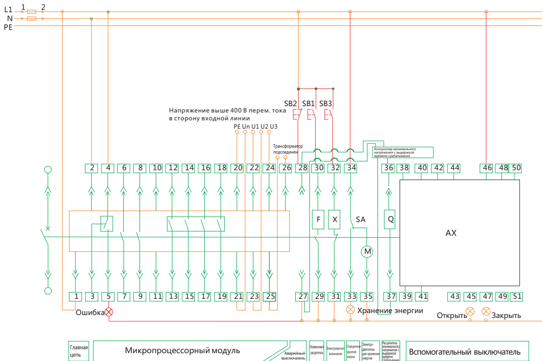
Вторичная схема микропроцессорного блока типа 3М NA1-2000X~6300X (с распределителем минимального напряжения с задержкой)
