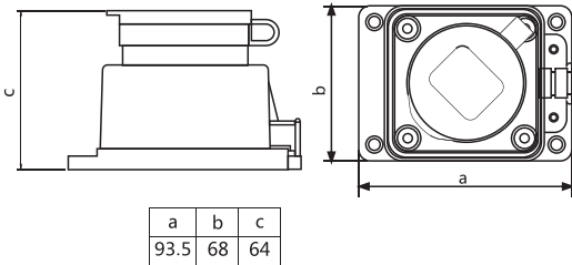
Розетка настенная с заглушкой каучук 2P+PE 16A 220B IP44 ANDELI
