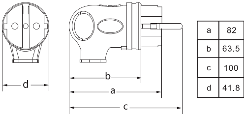
Вилка с ручкой каучук AM-K07 2P+PE 16A 220B IP44
