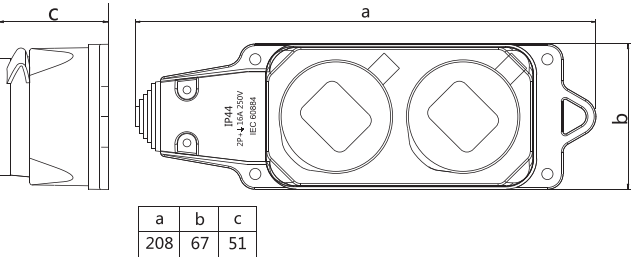
Розетка двухместная с заглушками каучук 2P+PE 16A 220B IP44 (ANDELI)
