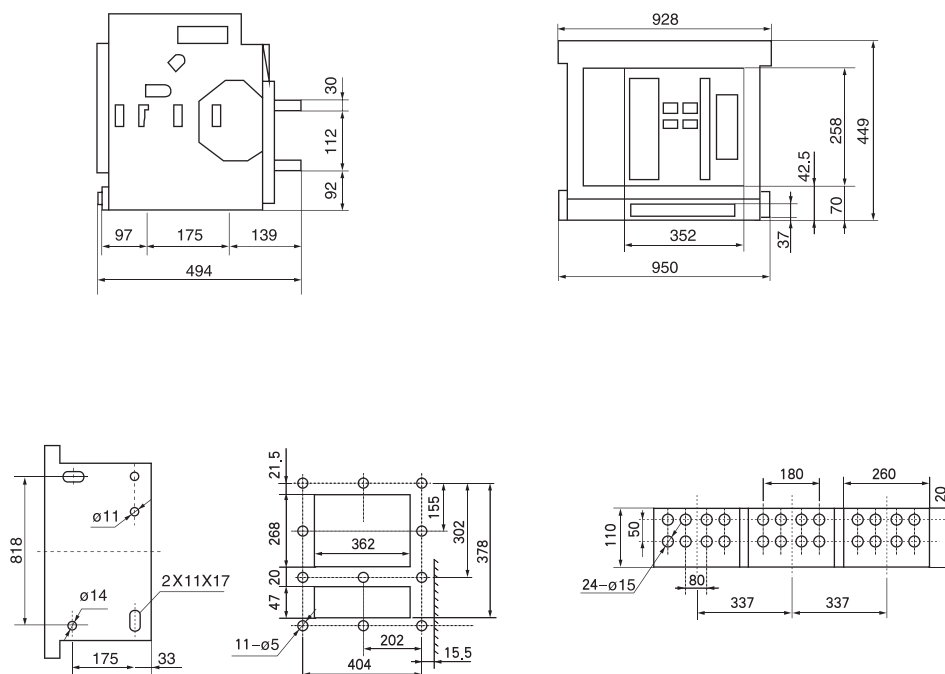
AW45-6300 ВЫДВИЖНОЙ (3-pole)
