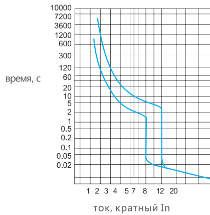
время-токовая характеристика AM1-1250
