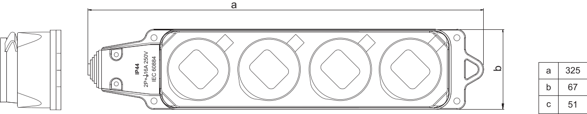
Розетка четырехместная с заглушками каучук AM-K06 2P+PE 16A 220B IP44 (ANDELI)
