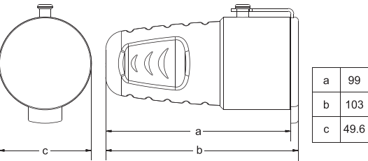
Розетка переносная с заглушкой каучук 2P+PE 16A 220B IP44 ANDELI
