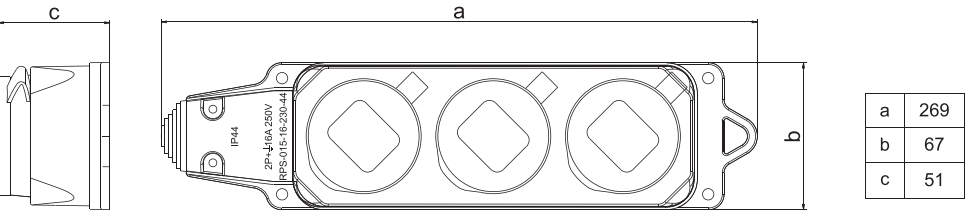
Розетка трехместная с заглушками каучук 2P+PE 16A 220B IP44 ANDELI
