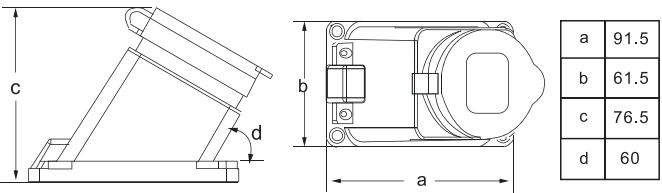
Розетка наклонная с заглушкой каучук AM-K08 2P+PE 16A 220B IP44
