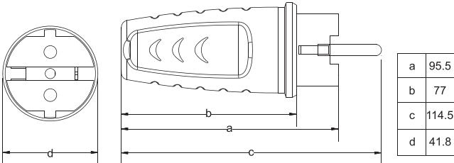
Вилка прямая каучук 2P+PE 16A 220B IP44 ANDELI
