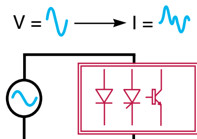
Рис. 16. Нелинейные потребители создают гармоники
