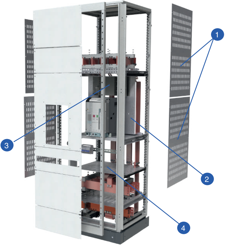
Элементы разделения функциональных блоков FBV, FBH
