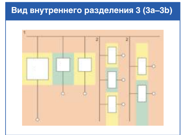
Отделение сборных шин от всех функциональных блоков
