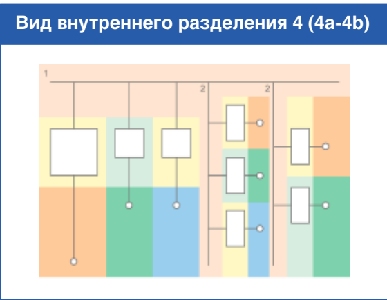
Отделение выводов для внешних проводников и внешних проводников от функциональных блоков
