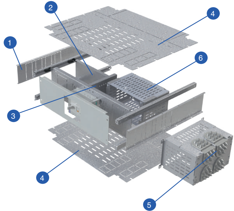
Элементы разделения функциональных блоков FBV, FBH
