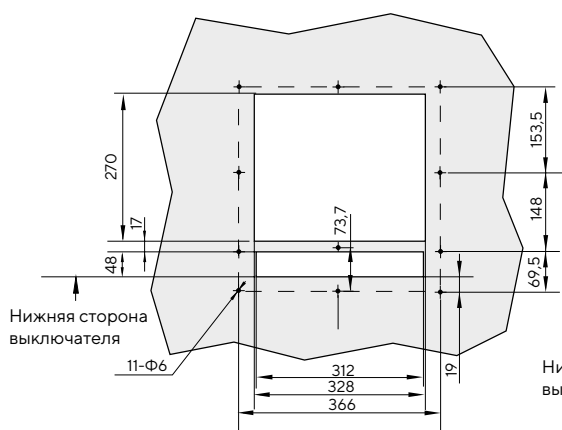
Выдвижной
