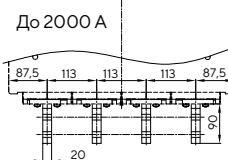
Вид Б (вертикальные выводы)
