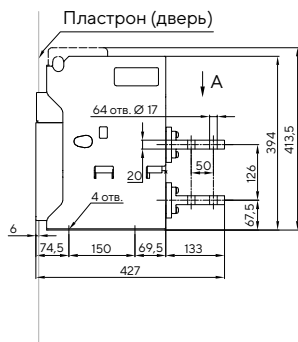
Вид сбоку Вариант 2. Вертикальные выводы
