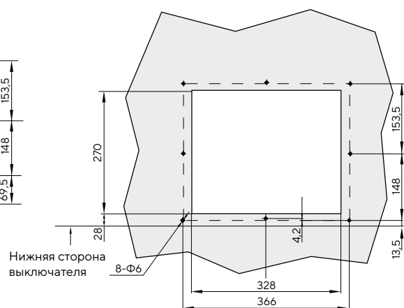
Стационарный
