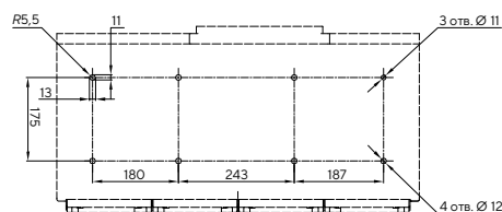
Расположение крепежных отверстий (вид снизу)
