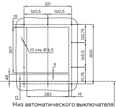
Расположение крепежных отверстий (вид снизу)
