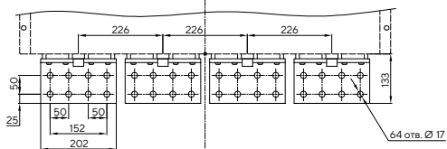
Вид А (горизонтальные выводы)
