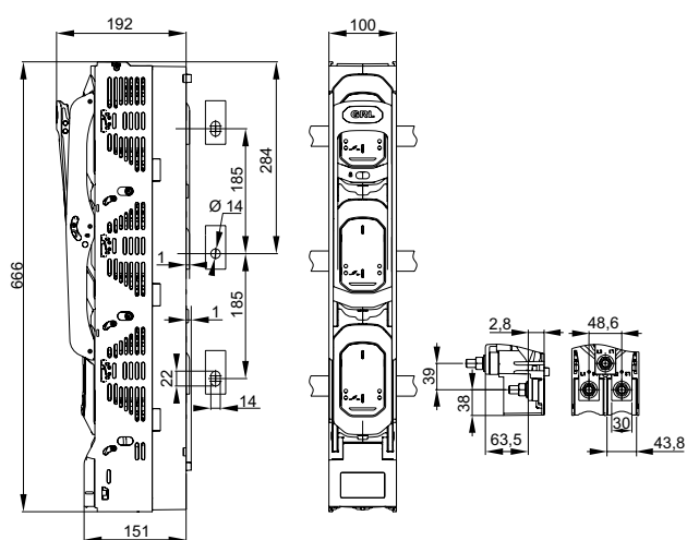
ПВР-1 250-630 А
