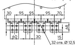
Вид А (горизонтальные выводы)
