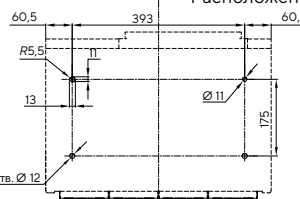
Расположение крепежных отверстий (вид снизу)
