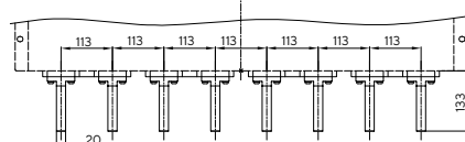
Вид Б (вертикальные выводы)
