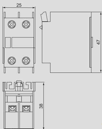
ПКИ-11, ПКИ-20
