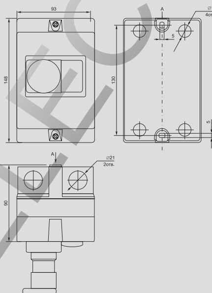
Защитная оболочка IP54
