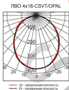
ЛВО 4x18-CSVT/OPAL
