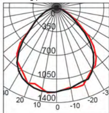
Alumogips-15/ice 295x595
