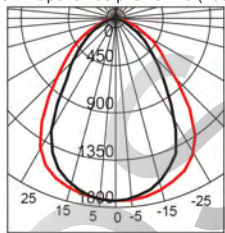
CSVT Operlux-38/prisma/R-3 (236)
