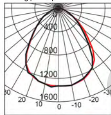
Alumogips-30/prisma 295x1195
