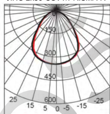
ЛПО 2x36-CSVT/PRISMA-R
