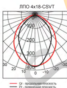
ЛПО 4x18-CSVT
