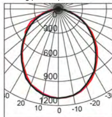
Alumogips-30/opal 295x1195
