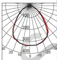
ЛВО 4x18-CSVT/PRISMA
