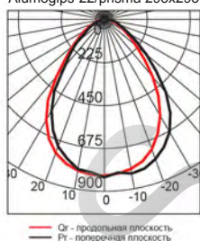
Alumogips-22/prisma 295x295
