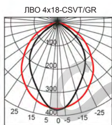
ЛВО 4x18-CSVT/GR
