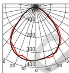
ЛПО 4x18-CSVT/ICE-R
