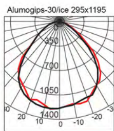
Alumogips-30/ice 295x1195
