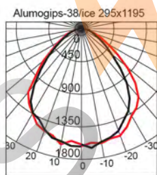
Alumogips-38/ice 295x1195
