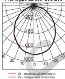
Alumogips-22/opal 295x295
