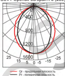
CSVT Operlux-38/opal/R-3 (236)
