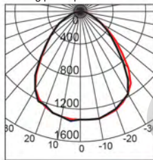
Alumogips-15/prisma 295x595
