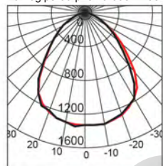
Alumogips-60/prisma 595x1195
