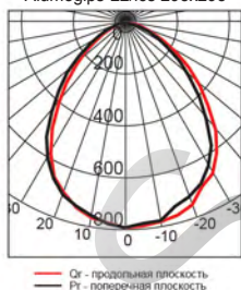
Alumogips-22/ice 295x295
