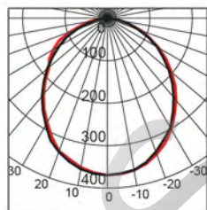
ЛПО 4x18-CSVT/OPAL-R
