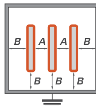
Щитовое устройство с изолированными шинами
