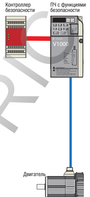
Схема безопасности с ПЧ с функцией безопасности
