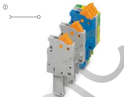
17,5 А, штекер, подключение вертикальное, для монтажа по месту
