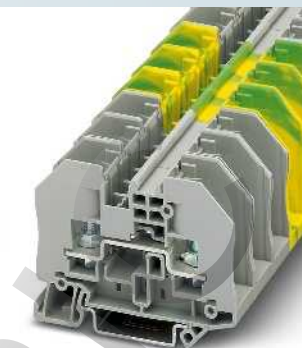
41 А, проходная клемма, открытая
