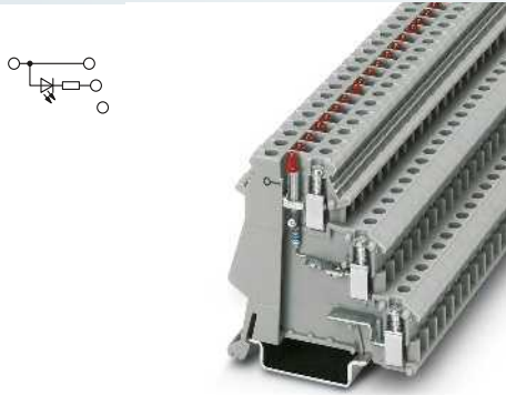
2,5 (4) мм 2 , 26 А, трехпроводная клемма со световым индикатором
