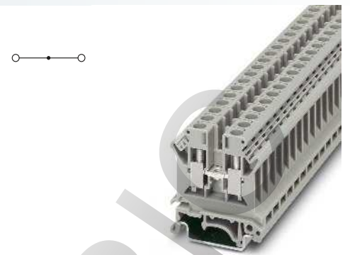
6 (10) мм 2 , 57 A, проходная клемма
