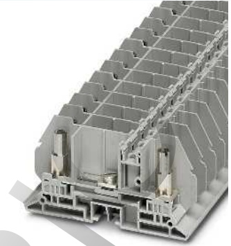
10 (10) мм 2 , 50 А, клемма с размыкателем для измерительного трансформатора, для непосредственного монтажа
