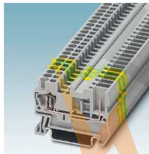
Проходные, многопроводные и многояру- сные клеммы, а также заземляющие клеммы с пружинными зажимами 2,5 мм 2 ... 4 мм 2 ...
