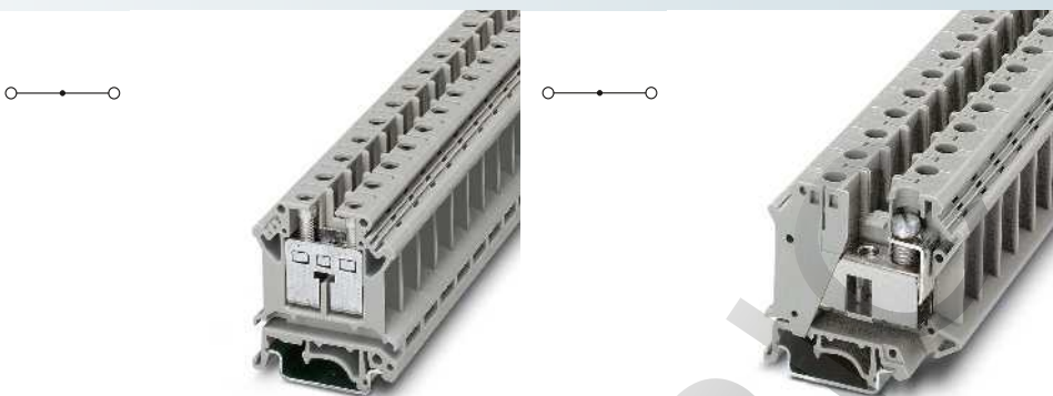
16 (25) мм 2 , 101 А, проходная клемма
