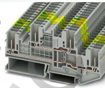
22 А, двухъярусные клеммы
