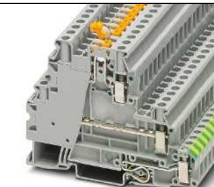
36 А, многоярусная клемма с ножевым размыкателем и контактом PE
