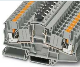
5 А, 1000 В, диодная клемма, той же формы
