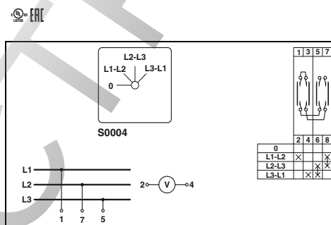
2,5 (2,5) мм 2 , 20 А, переключатель вольтметра с положением 0
