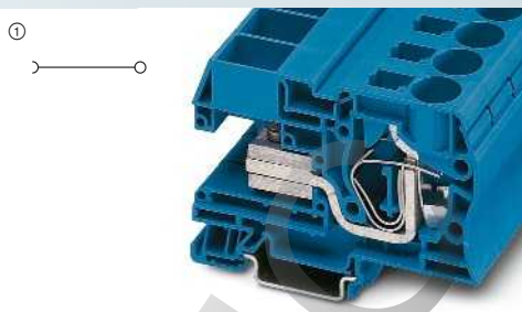
125 A, клемма с размыкателем N
