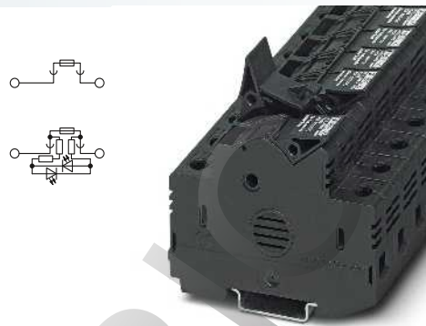
25 (25) мм 2 , 30 А, 1000 В, клемма для предохранителя 10,3 x 38 мм
