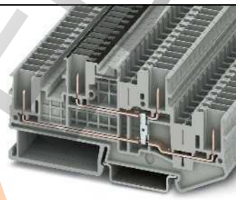
22 А, двухъярусная клемма с объединением потенциалов
