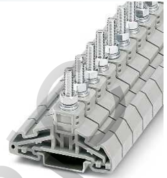
35 (35) мм 2 , 125 А, М6 болтовая клемма
