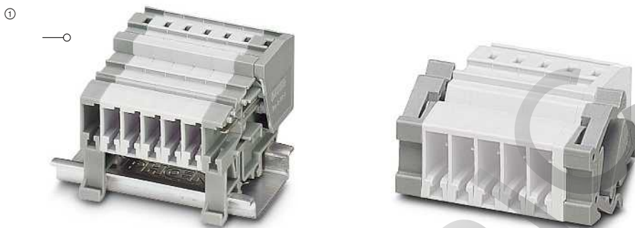
32 А, Розетки COMBI для крепления на DIN рейке
