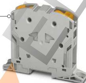
232 А, проходная клемма, для прямого монтажа
