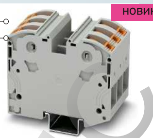
125 А, клеммный блок
