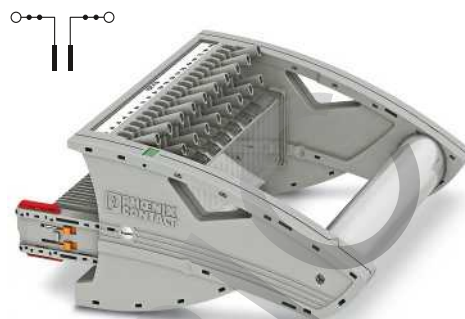
24 А, контрольная крышка, переключки в соответствии со схемой, кодировка VDE
