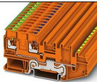
2,5 (4) мм 2 , 20 А, вводная клемма с заземляющим контактом
