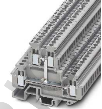
2,5 (4) мм 2 , 24 А, двухъярусная клемма с внутренним соединением ярусов
