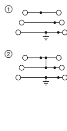
28 А, трехъярусная клемма с основанием PE
