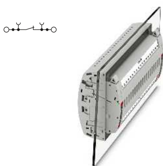
6 (10) мм 2 , 30 А, базовый блок, кодировка VDE тип H19
