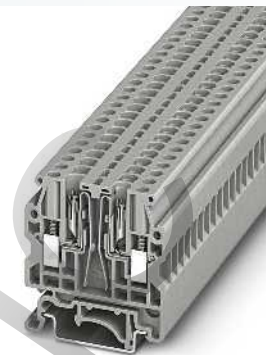
4 (6) мм 2 , клемма с размыкателем для измерительных трансформаторов
