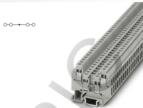
1,5 (1,5) мм 2 , 16 А, проходная клемма, 4 контакта
