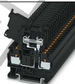
6,3 А, клемма для стеклянных предохранителей 5 x 20 мм, 2 функциональных отверстия
