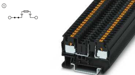
15 А, клеммы для плоских предохранителей типа F
