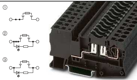
30 А, клеммы для плоских предохранителей тип С
