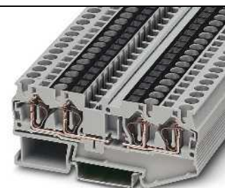
37 А, клемма с разрывом цепи, 4 контакта
