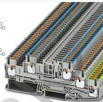
30 А, трехъярусная клемма с зоной разделения и заземляющим контактом
