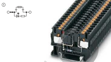
15 А, клеммы для плоских предохранителей типа F, с индикацией
