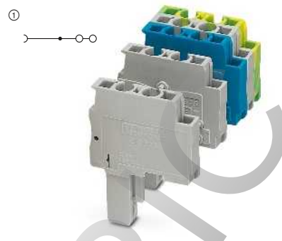
24 А, штекер, два контакта в направлении проводника, для монтажа по месту
