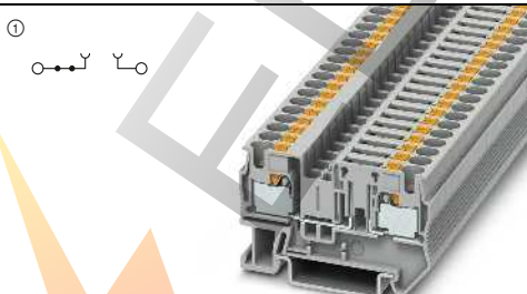
20 А, клемма с разрывом цепи
