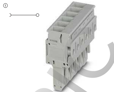
41 А, штекер, подключение в направлении проводника
