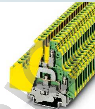
4 (4) мм 2 , двухъярусная заземляющая клемма
