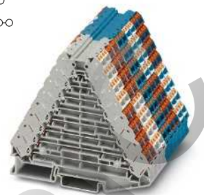
8 А, распределительные клеммы, 32 контакта
