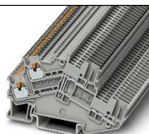
16 А, двухъярусная клемма с перемычкой между ярусами
