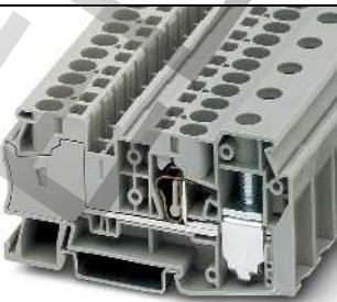
125 A (винтовой зажим), распределительная клемма, 4 отвода 10 мм 2
