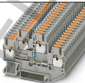
20 А, двухъярусная клемма с резистором
