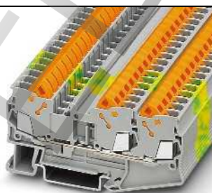
24 А, проходная клемма, 3 контакта
