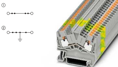
30 А, проходная клемма
