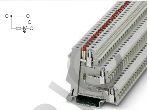
2,5 (4) мм 2 , 26 А, трехпроводная клемма со световым индикатором
