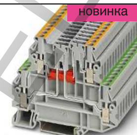
16 А, двухъярусная клемма с двумя разделительными зонами
