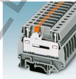
Клеммы для поперечного переключения UGSK/S Стр. 421
