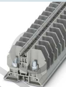
10 (10) мм 2 , 57 А, проходная клемма, для непосредственного монтажа
