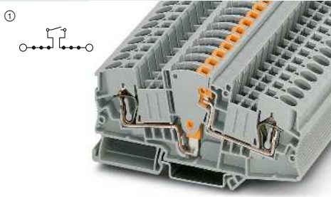
30 А, Клемма для измерит. трансформаторов
