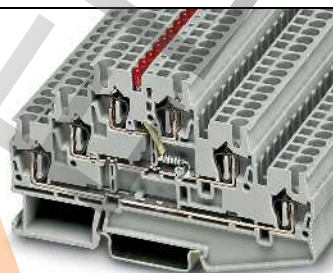
28 А, трехъярусная клемма со световым индикатором
