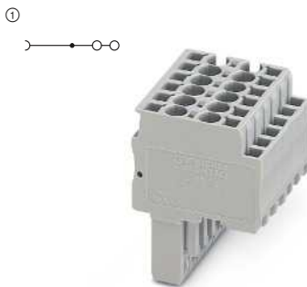
24 А, штекер, два контакта в направлении проводника
