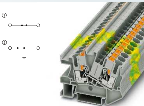
41 А, проходная клемма
