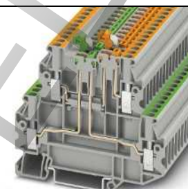
16 А, двухъярусная клемма с ножевыми размыкателями на каждом ярусе и полыми винтами для щупа тестера
