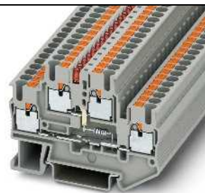
24 А, двухъярусная клемма со световым индикатором
