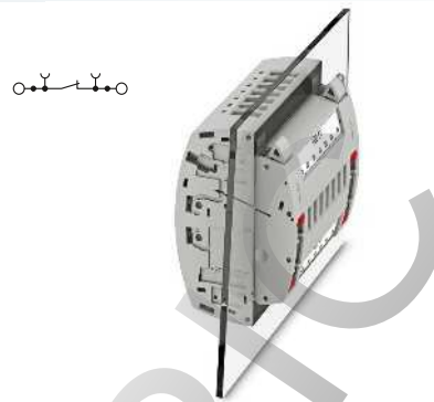
6 (10) мм 2 , 30 А, базовый блок, кодировка VDE тип A7
