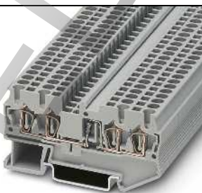
0,5 А, диодные клеммы, 1N 4007 (1300 В/0,5 А), 4 контакта
