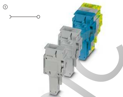
41 А, штекер, подключение в направлении проводника, для монтажа по месту
