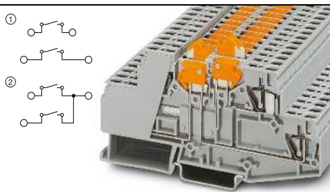
16 А, двухъярусная клемма с ножевым размыкателем на каждом ярусе
