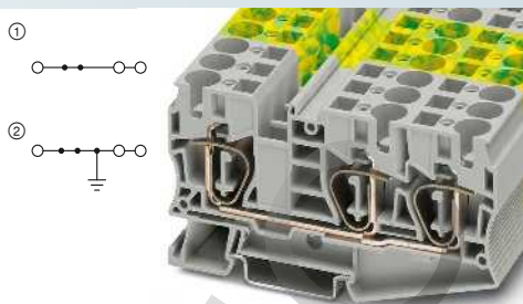
70 А, проходные клеммы, 3 контакта
