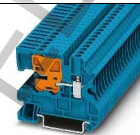
24 А, клемма с размыкателем N
