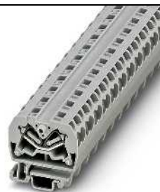
30 А, проходная клемма, боковой ввод, 4 контакта
