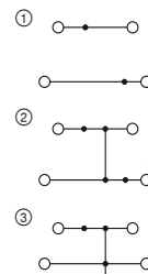
17,5 А, двухъярусные клеммы
