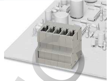
32 А, разъем на плату, вертикальное направление подключения
