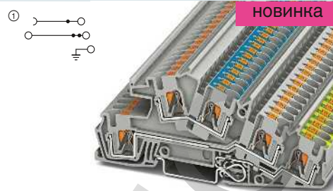
32 А, трехъярусная клемма, 2 фазных провода L, 1 PE
