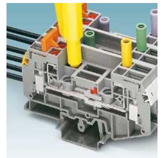
Клеммы с размыкателями для измерительных трансформаторов URTK 6 Стр. 427
