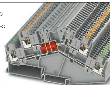
16 А, двухъярусная клемма с двумя зонами разрыва цепи
