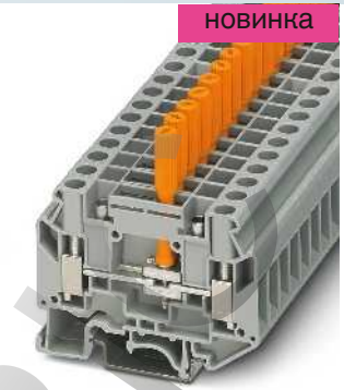
6 (10) мм 2 , 57 А, клемма с размыкателем
