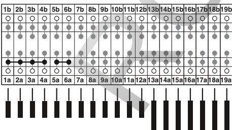
Тестовый штекер типа I19
