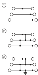
28 А, трехъярусная клемма
