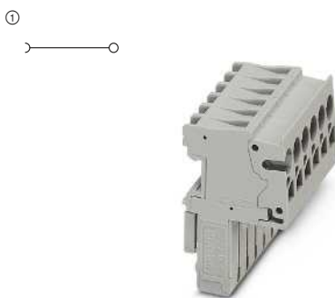
24 А, штекер, подключение под прямым углом к направлению проводника
