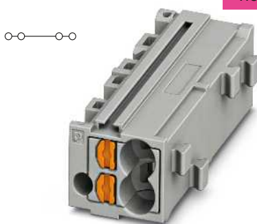
22 А, отдельный элемент, 4 контакта
