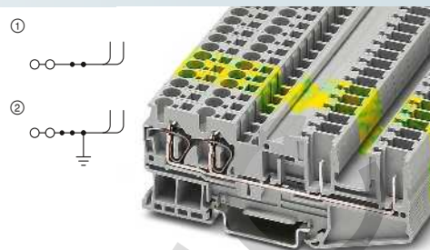
32 А, проходная клемма, 4 контакта
