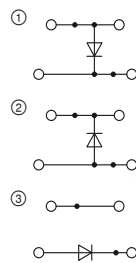
26 А, диодные двухъярусные клеммы, 1N 4007 (1300 В/0,5 А)
