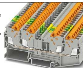
24 А, проходная клемма, 4 контакта
