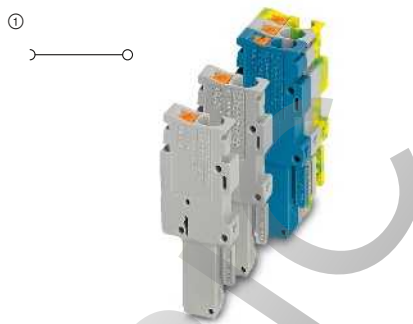
24 А, штекер, подключение в направлении проводника, наборные элементы
