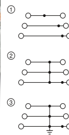
15 А, многоярусная клемма, 6 контактов
