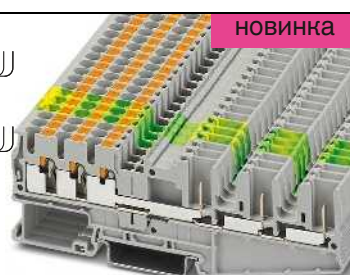
24 А, проходная клемма, 6 контактов
