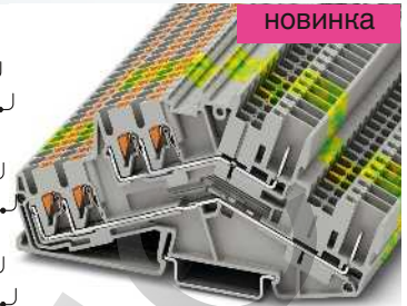
22 А, двухъярусная клемма, угловая конструкция
