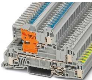
4 (4) мм 2 , 30 А, трехъярусная клемма, 1 проходной ярус L, 1 ярус N с размыканием, 1 PE
