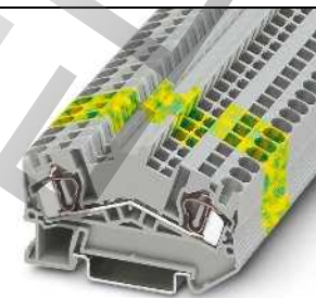
38 А, проходная клемма
