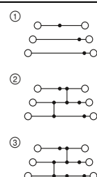
24 А, многоярусная клемма
