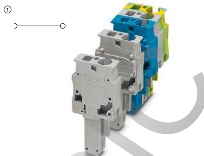
32 А, штекер, подключение вертикальное, для монтажа по месту
