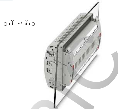
6 (10) мм 2 , 30 А, базовый блок, кодировка VDE тип I19
