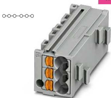
22 А, отдельный элемент, 6 контактов
