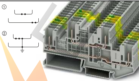
22 А, двухъярусные клеммы
