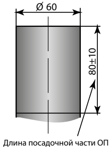
Рис. А-2 Стандартное посадочное место торшерных ОП
