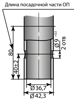
Рис. А-3 Стандартное посадочное место подвесных ОП
