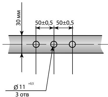
Рис. А-4 Стандартное посадочное место пржекторов
