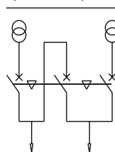
Принципиальная схема тройной блокировки ILK -3
