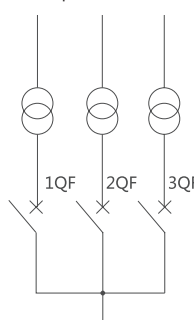
Принципиальная электрическая схема
