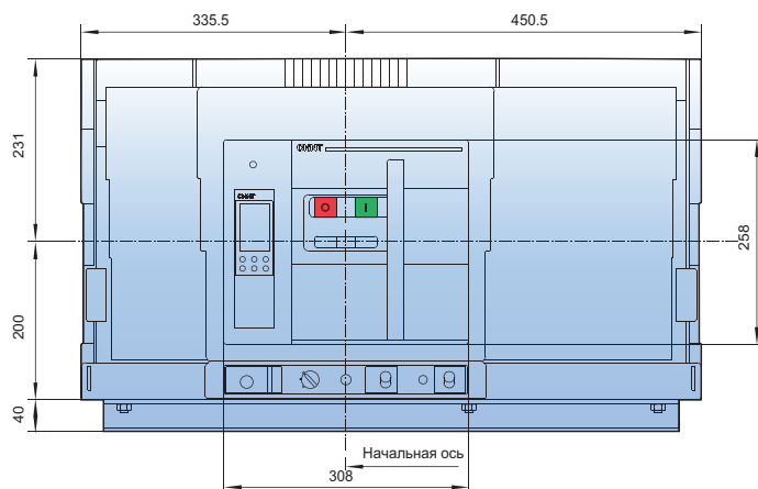
Вид спереди
