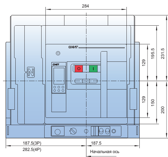
Вид спереди
