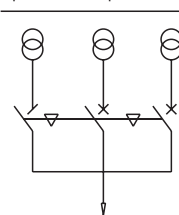
Принципиальная схема тройной блокировки ILK -4
