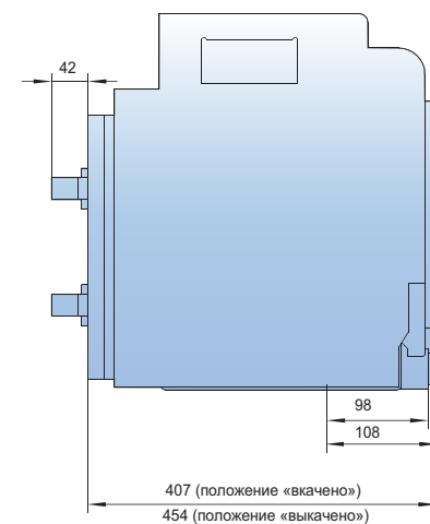
Вид сбоку
