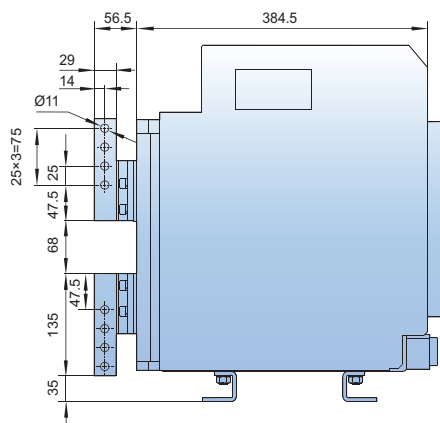
Вид сбоку
