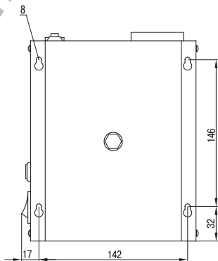
Рис 5. Задняя панель стабилизатора
