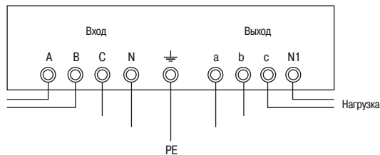
Рисунок 6. Схема подключения СНИЗ 3 кВА.
