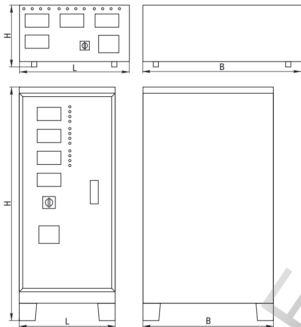
Рисунок 1. Габаритные размеры СНИЗ от 3 до 7,5 кВА
