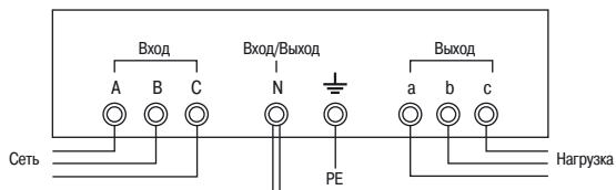
Рисунок 7. Схема подключения СНИЗ от 6 до 9 кВА.
