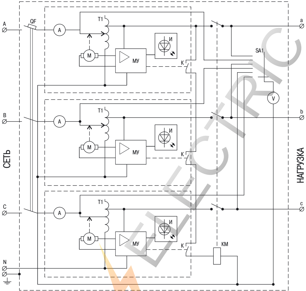
Рисунок 4а. СНИЗ 3, 6, 7,5 кВА
