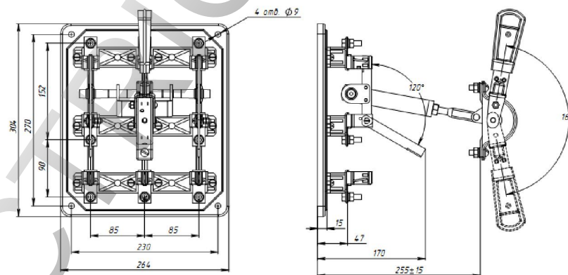
Рис. 1Б Разъединитель типа ПЦ с центральным приводом на ток 100 А
