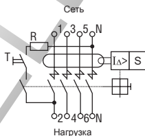
Рисунок 4. Схема электрическая принципиальная четырехполюсных ВД
