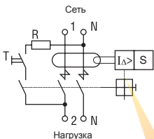
Рисунок 3. Схема электрическая принципиальная двухполюсных ВД
