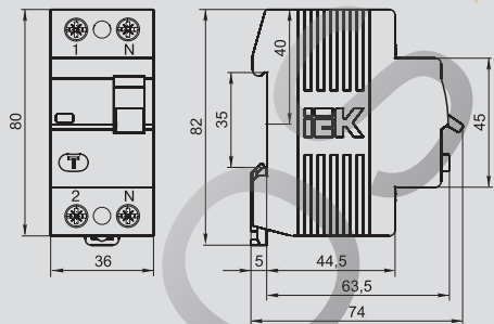
ВД1-63 тип А 2-полюсный
