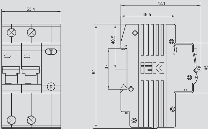
АД12, АД12М
