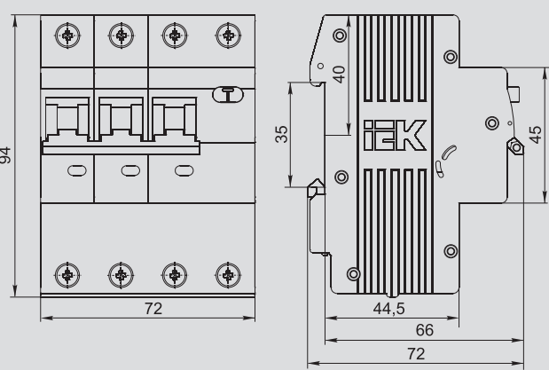
АВДТ34
