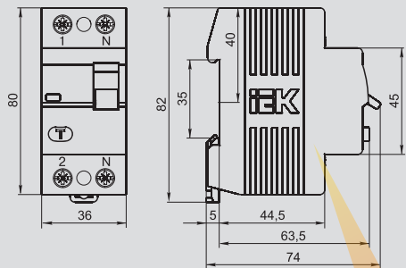
ВД1-63 2-полюсный
